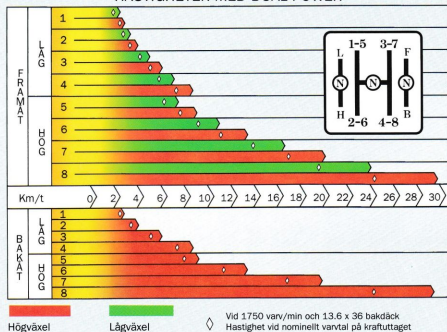
HASTIGHETER MED DUAL POWER
